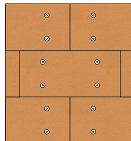
5 Stück/m 2
