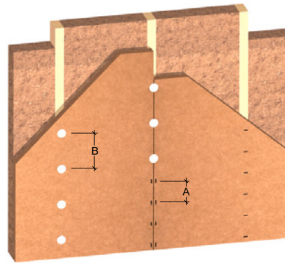
Großformatige Platten
